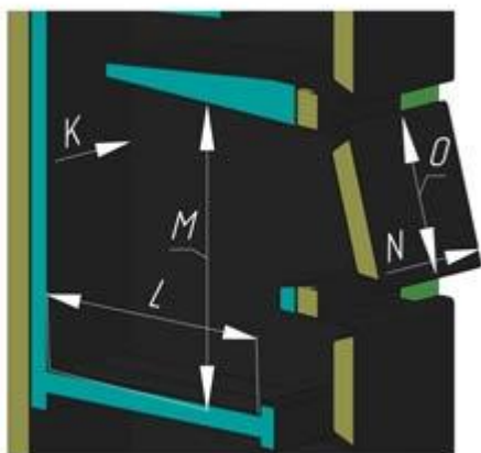
Рис 3. Размеры камеры сгорания котлов SAKOVICH YANO
