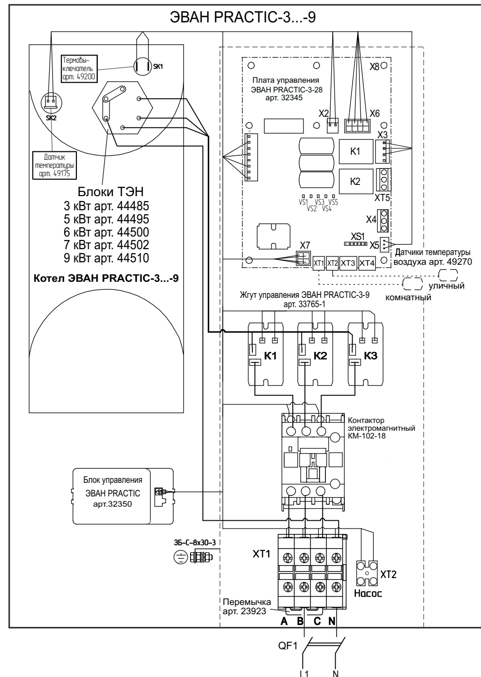
Рисунок 18. Схема подключения ЭВАН PRACTIC-3...-9 к сети 220В.
