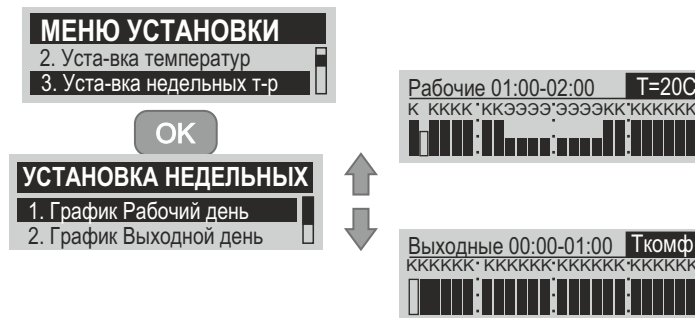
Рисунок 30. Настройка температурных режимов в недельном расписании.
