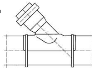
Рис. 15 Приклеиваемая накладная с раструбом
