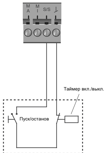
Рис. 24 Цифровой вход
