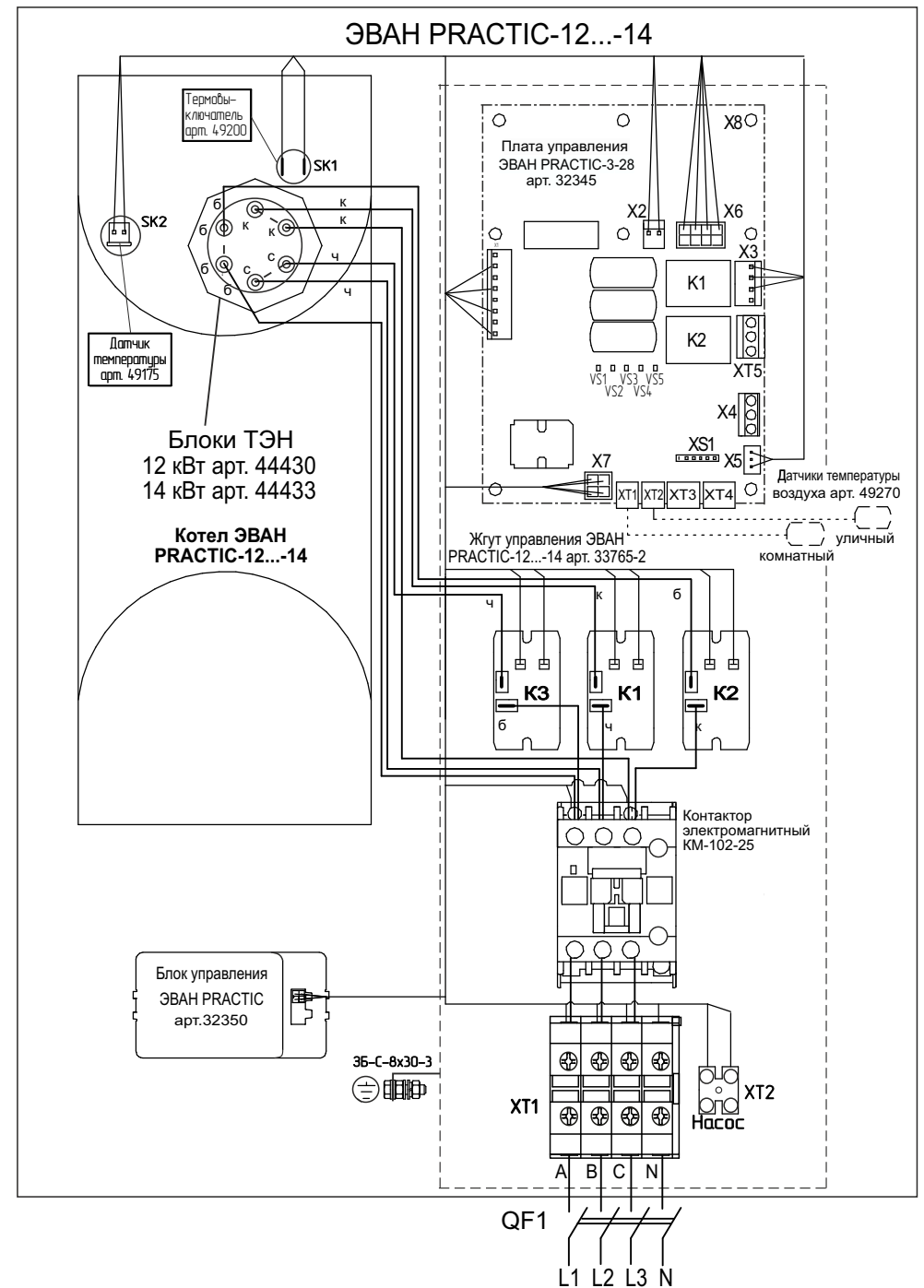
Рисунок 20. Схема подключения ЭВАН PRACTIC-12...-14.
