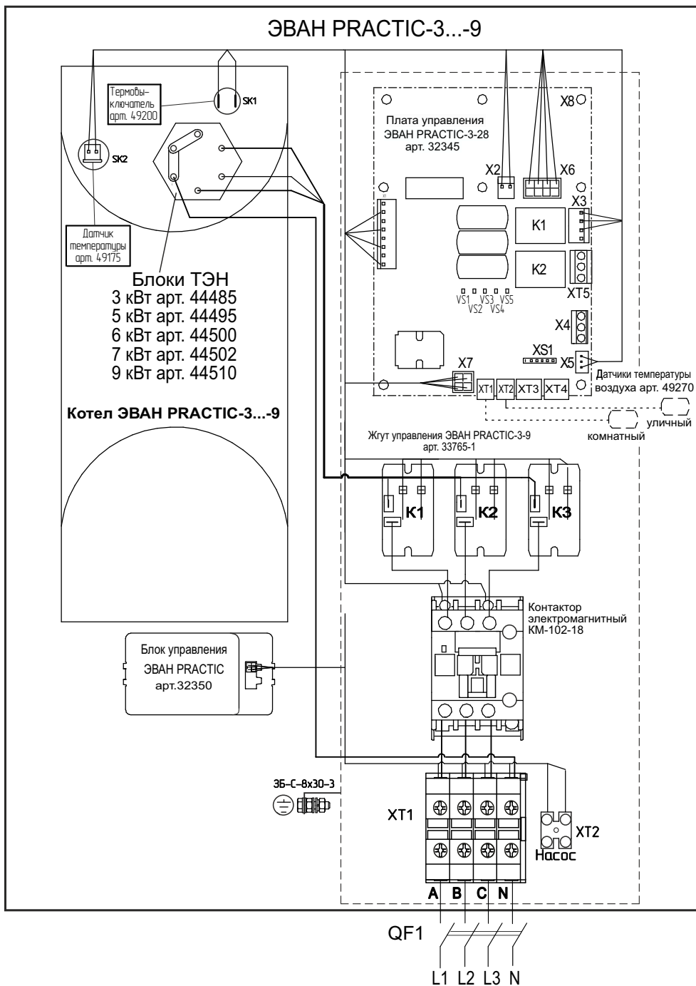
Рисунок 19. Схема подключения ЭВАН PRACTIC-3...-9 к сети 380В.
