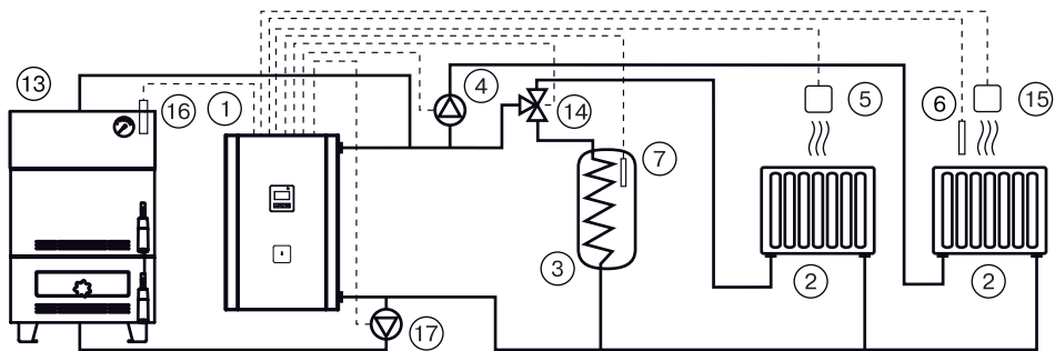
Рис.7 Упрощенная схема подключения миникотельной в режиме Отопление-ГВС
