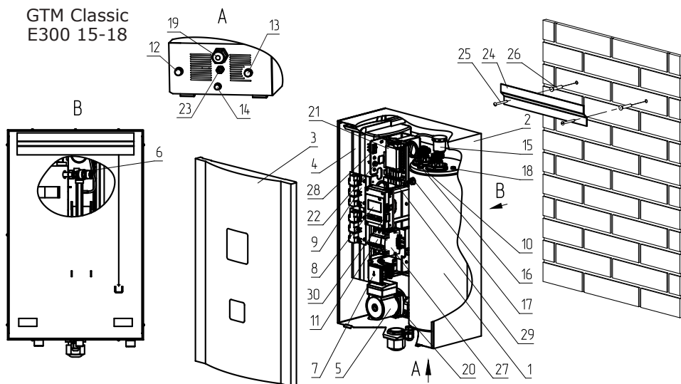
Рис.1 Конструкция миникотельной и способ её крепления к стене
