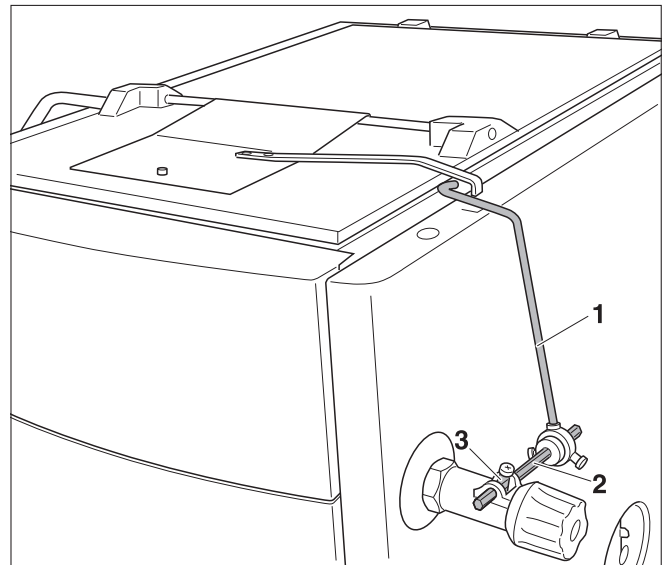
Рис. 9 Монтаж регулятора горения на котле типа K 32-1 SW 62
