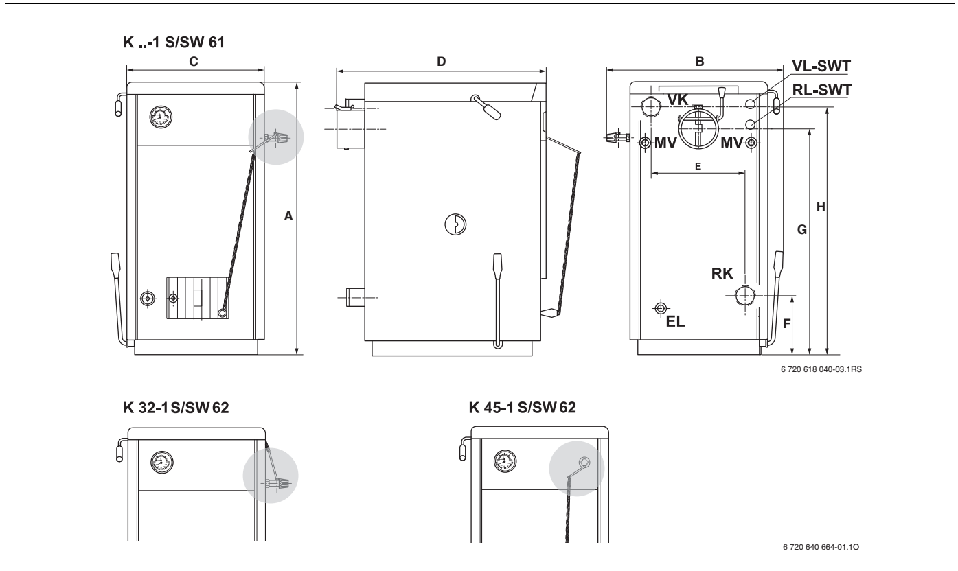
Рис. 3 Размеры и подключения
