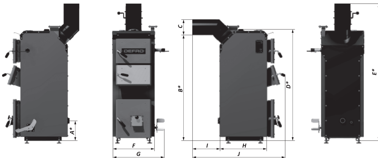
Рис. 1б. Основные размеры котлов OPTIMA KOMFORT в версии LUX .
