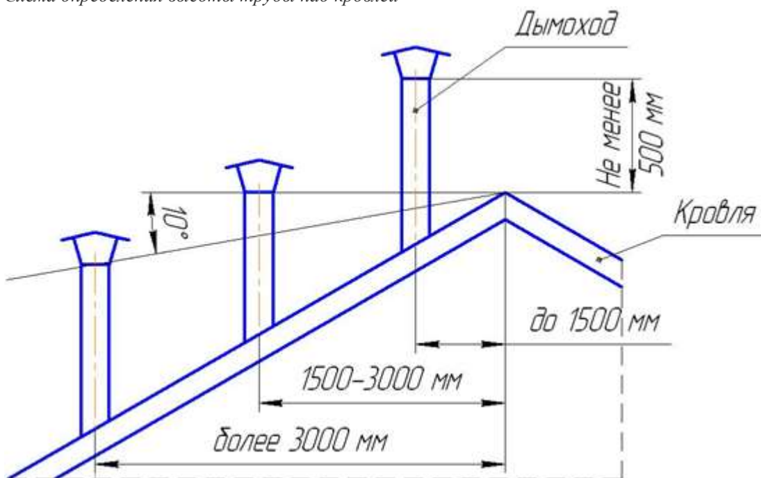
Рис.4 Схема определения высоты трубы над кровлей
