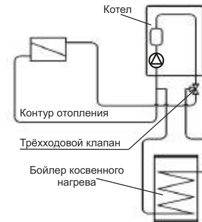
Рисунок 25. Гидравлическое подключение комплекта ГВС EVAN AQUA.
