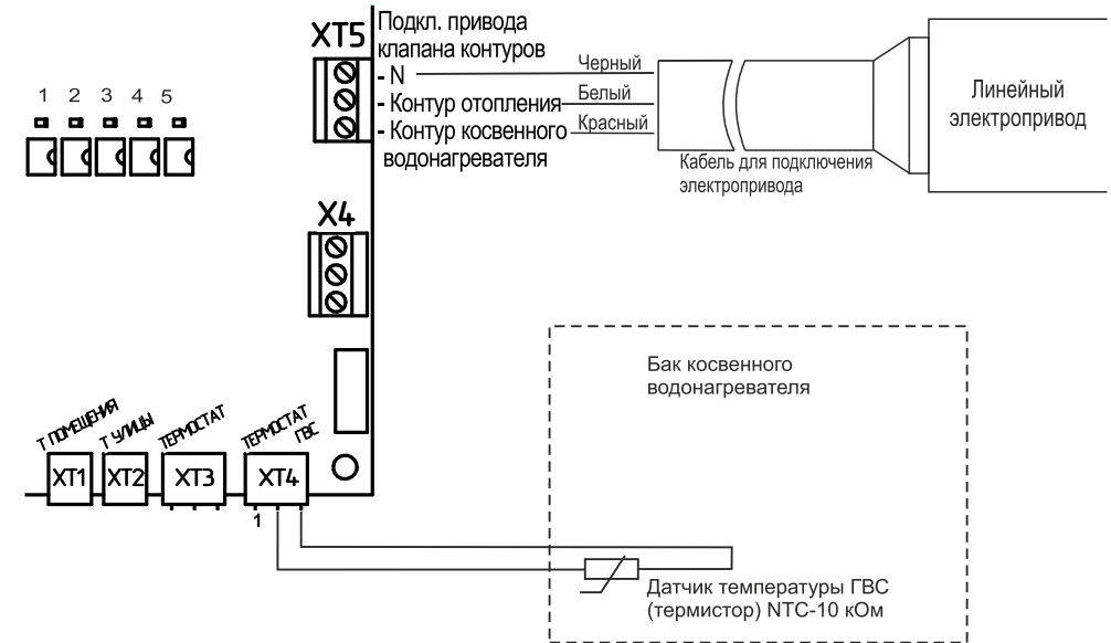
Рисунок 24. Электрическое подключение комплекта ГВС EVAN AQUA.
