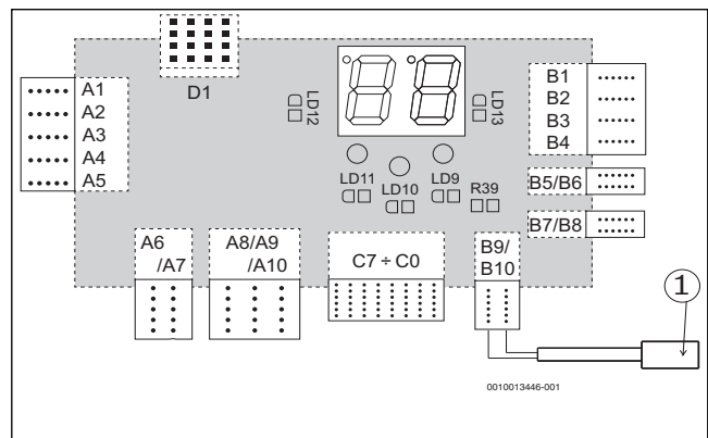
Fig. 1 Tilkobling av føleren på klemmene B9/B10
