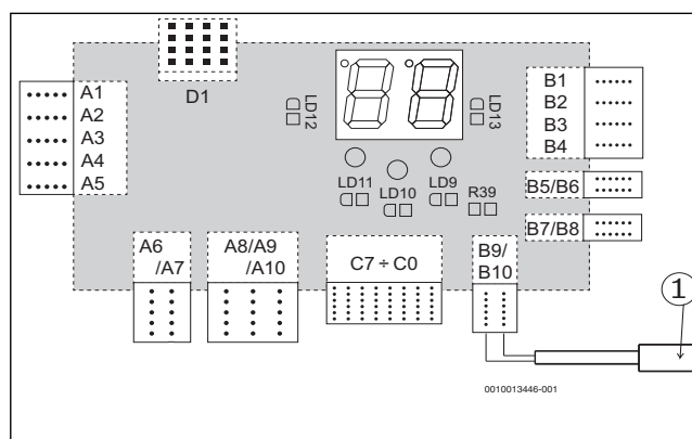
sl. 1 Priključivanje senzora na stezaljke B9/B10
