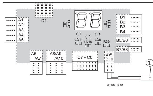
Фиг. 1 Свързване на датчика към клеми B9/B10
