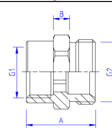
VTr. 592 NE Соединитель с переходом на «еврокonus» В-Н
