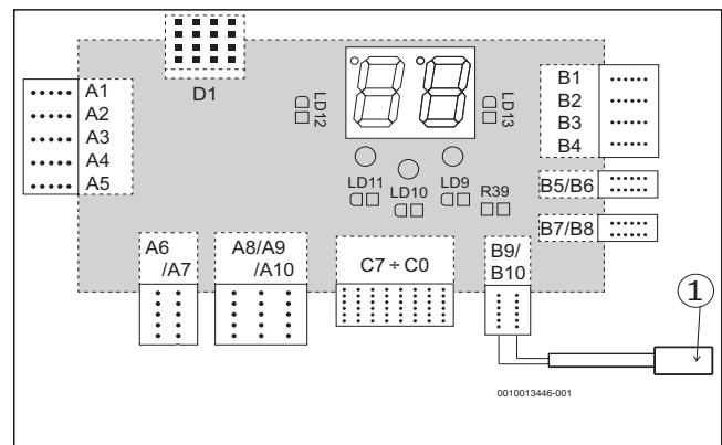
Сурет 1 Датчикті клеммаларға жалғау В9/В10
