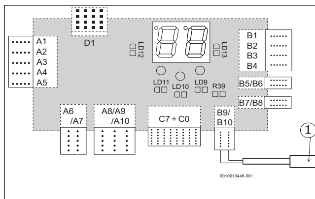
1. ábra Az érzékelő csatlakoztatása a B9/B10 csatlakozókapcsokhoz
