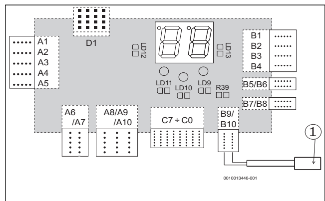
Obr. 1 Zapojení senzoru do svorek B9/B10
