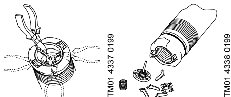
Рис. 14 Отрезание ножек клапана
