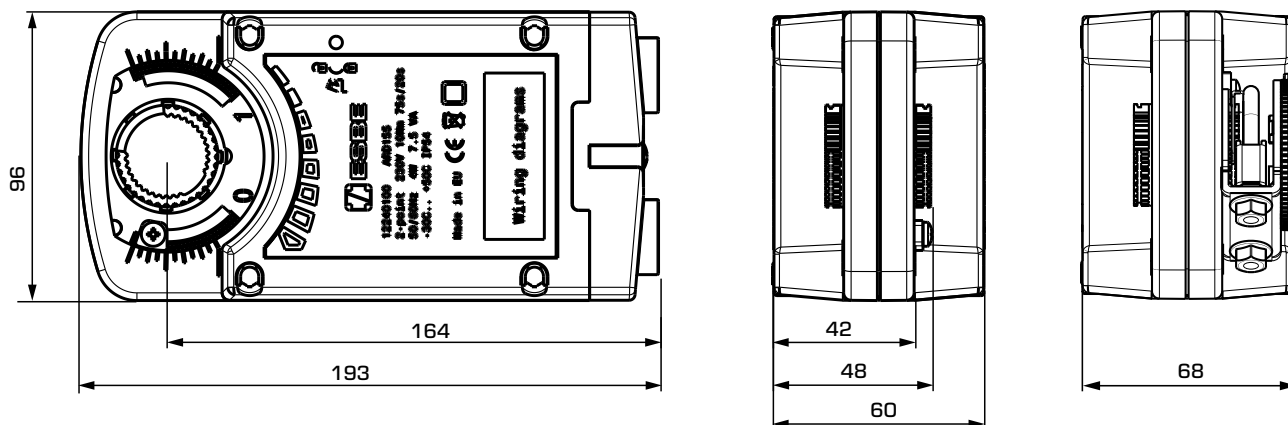
Привод серии ARD100
