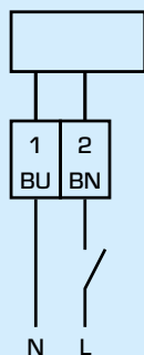
ARD155/ARD157 (2-точечный)
