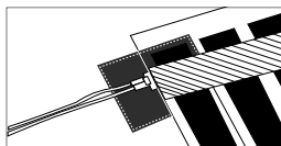
Изоляция места подключения с наружной стороны
