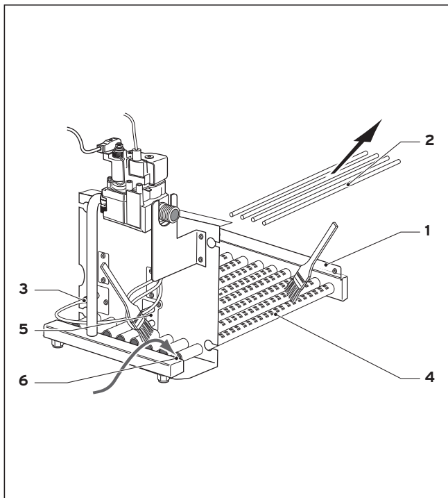
Slika 7.3 Čišćenje plamenika
