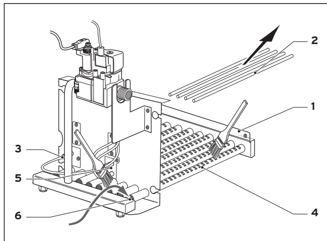
Fig. 7.3 Curățarea arzătorului
