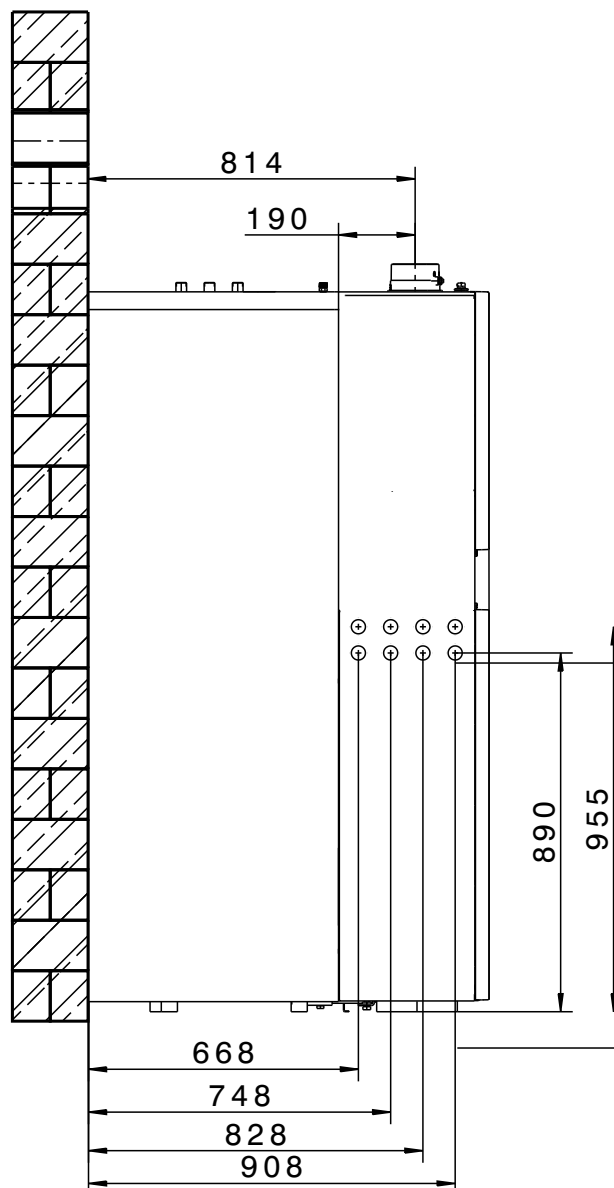
Вид сбоку CSZ-2R
