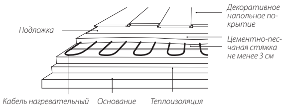
Схема укладки под ламинат, линолеум или ковролин в холодных помещениях
