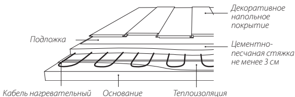
Схема укладки под ламинат, линолеум или ковролин
