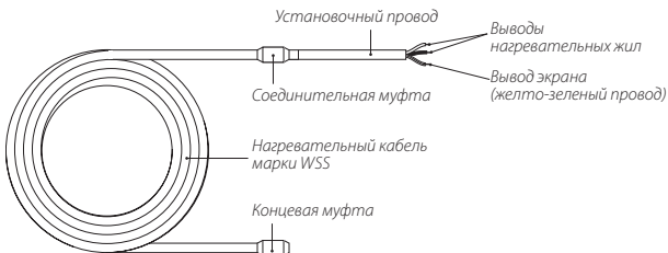
Конструкция кабеля нагревательного WSS
