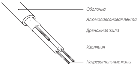
Конструкция кабеля нагревательного WSS
