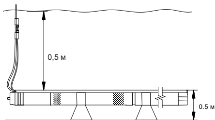
Рис. 8 Установка в горизонтальном положении
