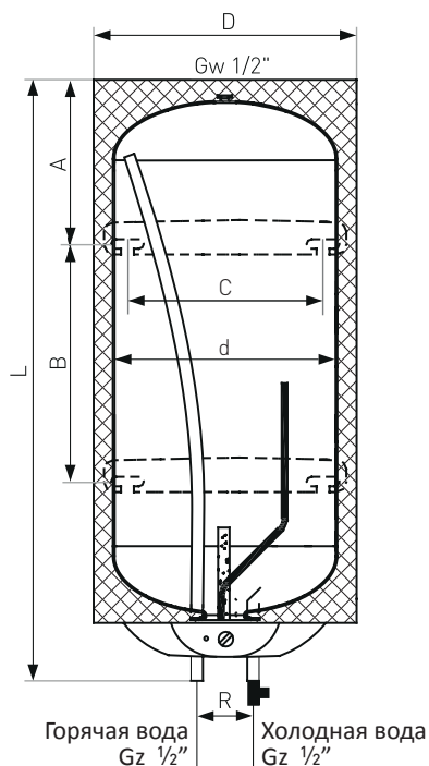
Схема водонагревателя для универсального монтажа:
