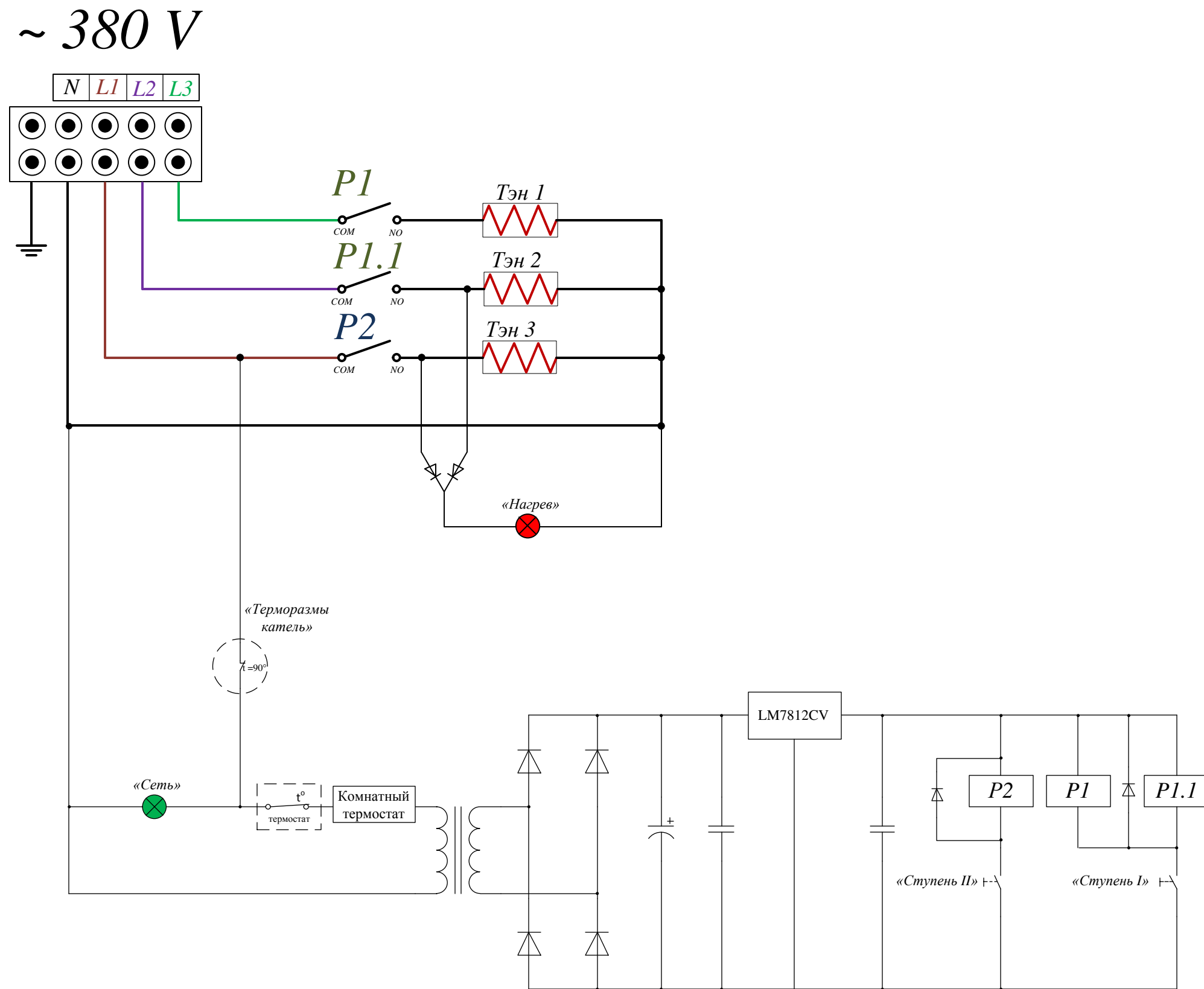
Рисунок 2 – Схема электрическая принципиальная для котлов «Есопот» на 380 В
