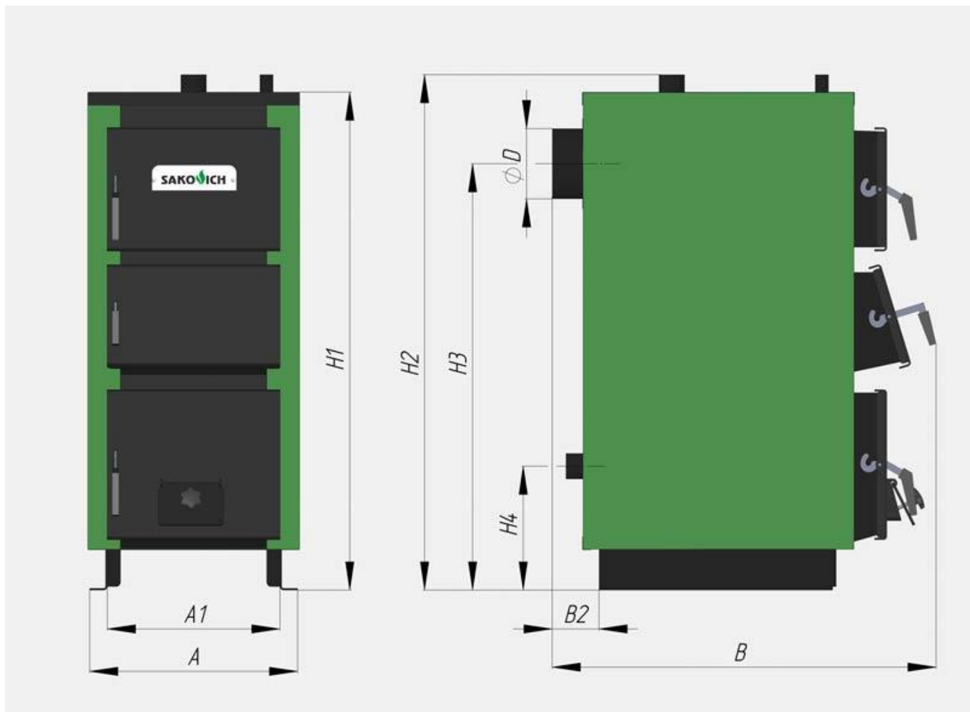
Рис 2. Размеры котлов SAKOVICH YANO
