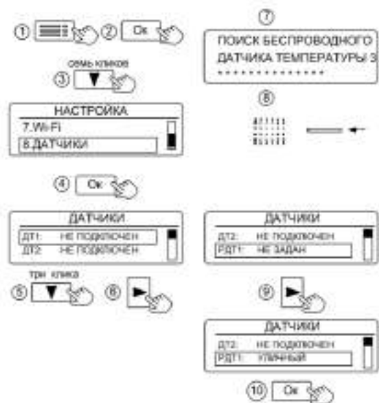
Рисунок 23. Настройка радиодатчиков
