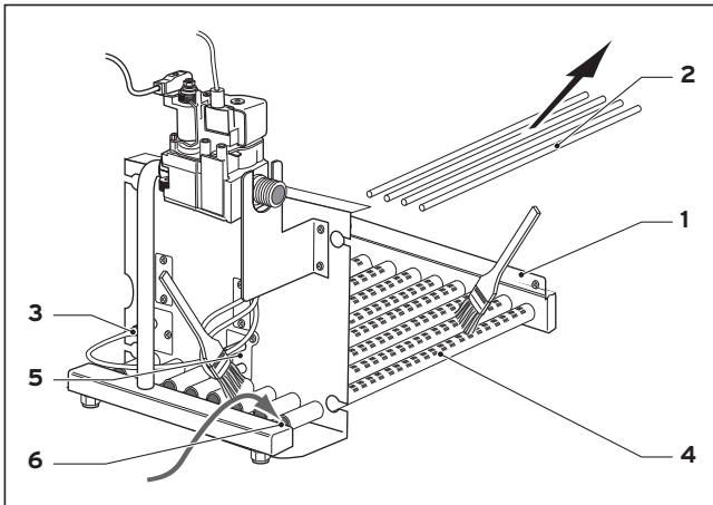
Рис. 7.3 Чистка горелки
