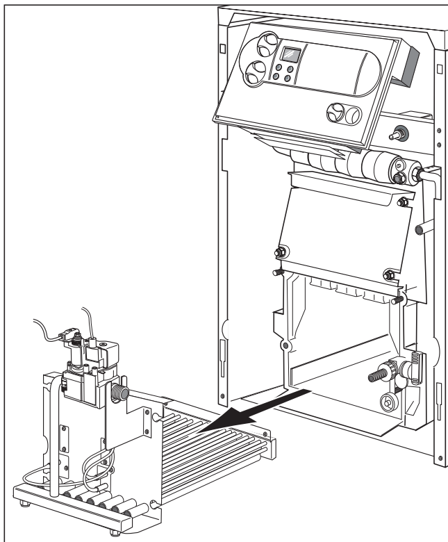
Slika 7.1 Demontaža plamenika
