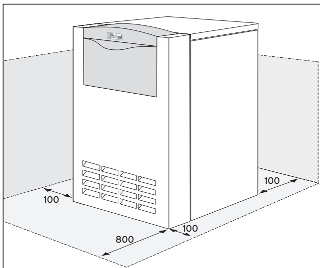
Slika 3.2: Minimalne udaljenosti
