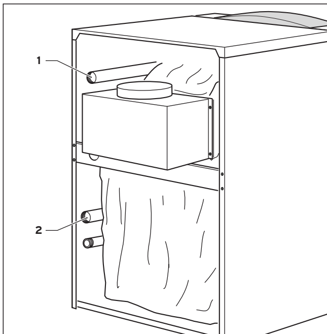
Sl. 4.1 Priključek s strani ogrevanja
