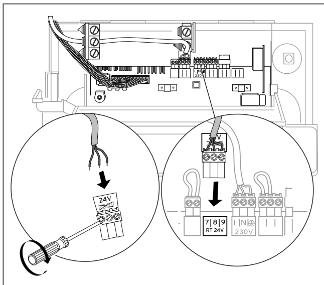
Sl. 4.7 Priključiti regulator na stezaljke 7-8-9
