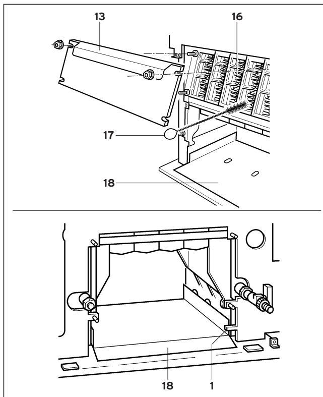
Рис. 7.2 Чистка теплообменника
