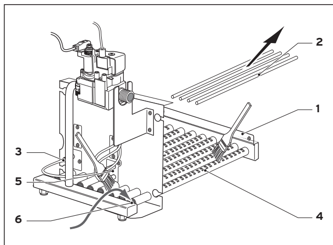
Fig. 7.3 Curățarea arzătorului
