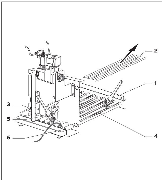
Slika 7.3 Čišćenje plamenika
