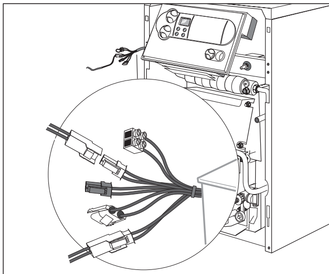
Slika 4.6: Priključivanje senzora
