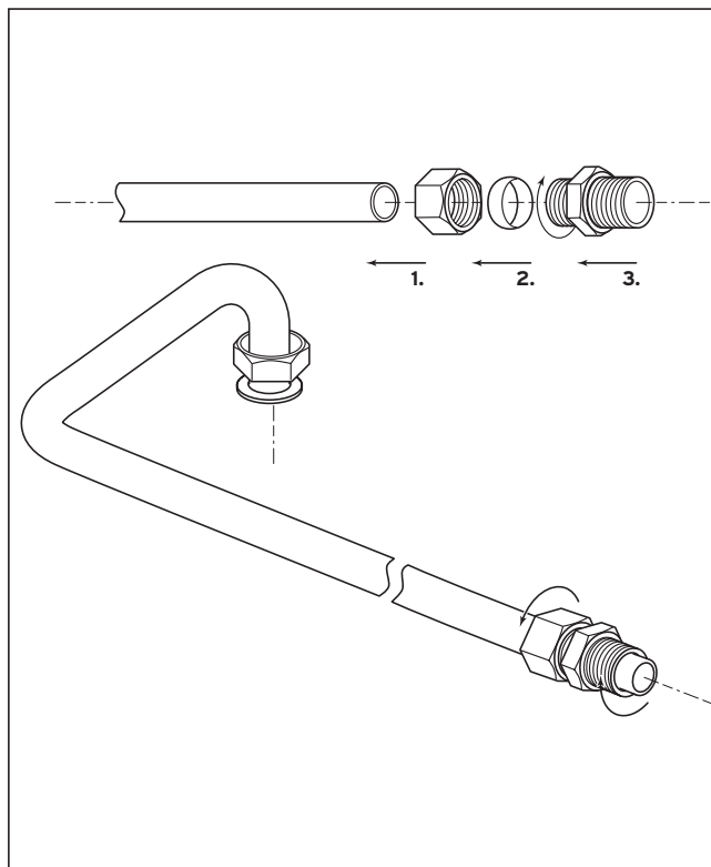
Slika 4.2: Plinski prikliučak
