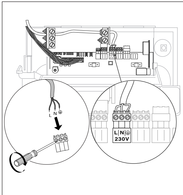
Slika 4.4: Priključivanje mrežnog voda
