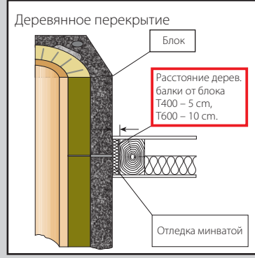
10.2 Деревянное перекрытие
