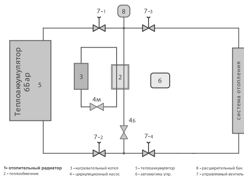
Рис.10. Схема с использованием теплоаккумулятора рассчитанным под высокие давления (6÷10 Бар). Давление в теплоаккумуляторе соответствует давлению в системе.
