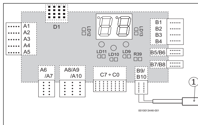
Фиг. 1 Свързване на датчика към клеми B9/B10
