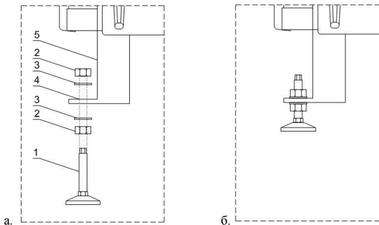
А) Способ монтажа ножек
