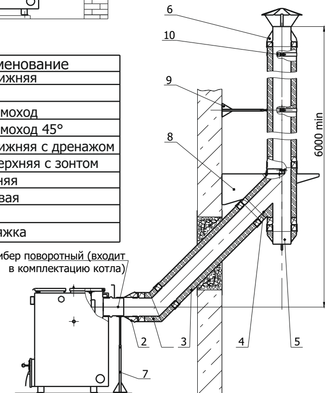
Рис.6е - Устройство дымоотведения с проходом через члену при помощи сэндвич колена 45° и сэндвич тройника 45° с заглушкой
