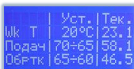
Рис. 23 – Внешний вид настроек таймеров и их отображение в меню Индикация
