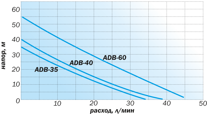
РАСХОДНО-НАПОРНЫЕ ХАРАКТЕРИСТИКИ НАСОСОВ при высоте всасывания от 0 до 0,5м и напряжении питания 220В
