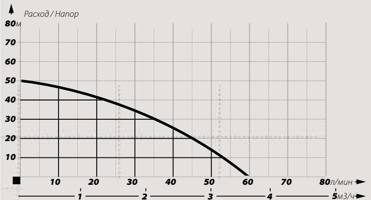
НАСОС AJ50/60 С АКЦЕССУАРАМИ
