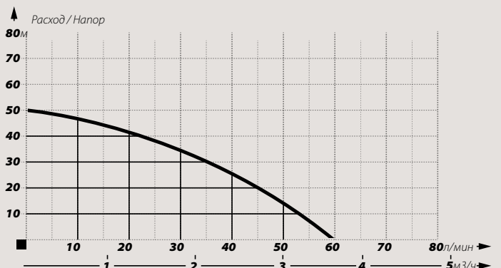
НАСОС JET 100 С АКЦЕССУАРАМИ
