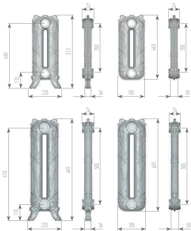
Размеры радиатора указаны без учета установленной арматуры и воздухоотводного клапана
