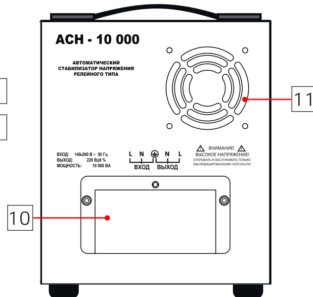
Задняя панель
