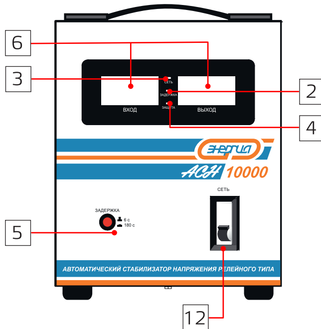
Лицевая панель
