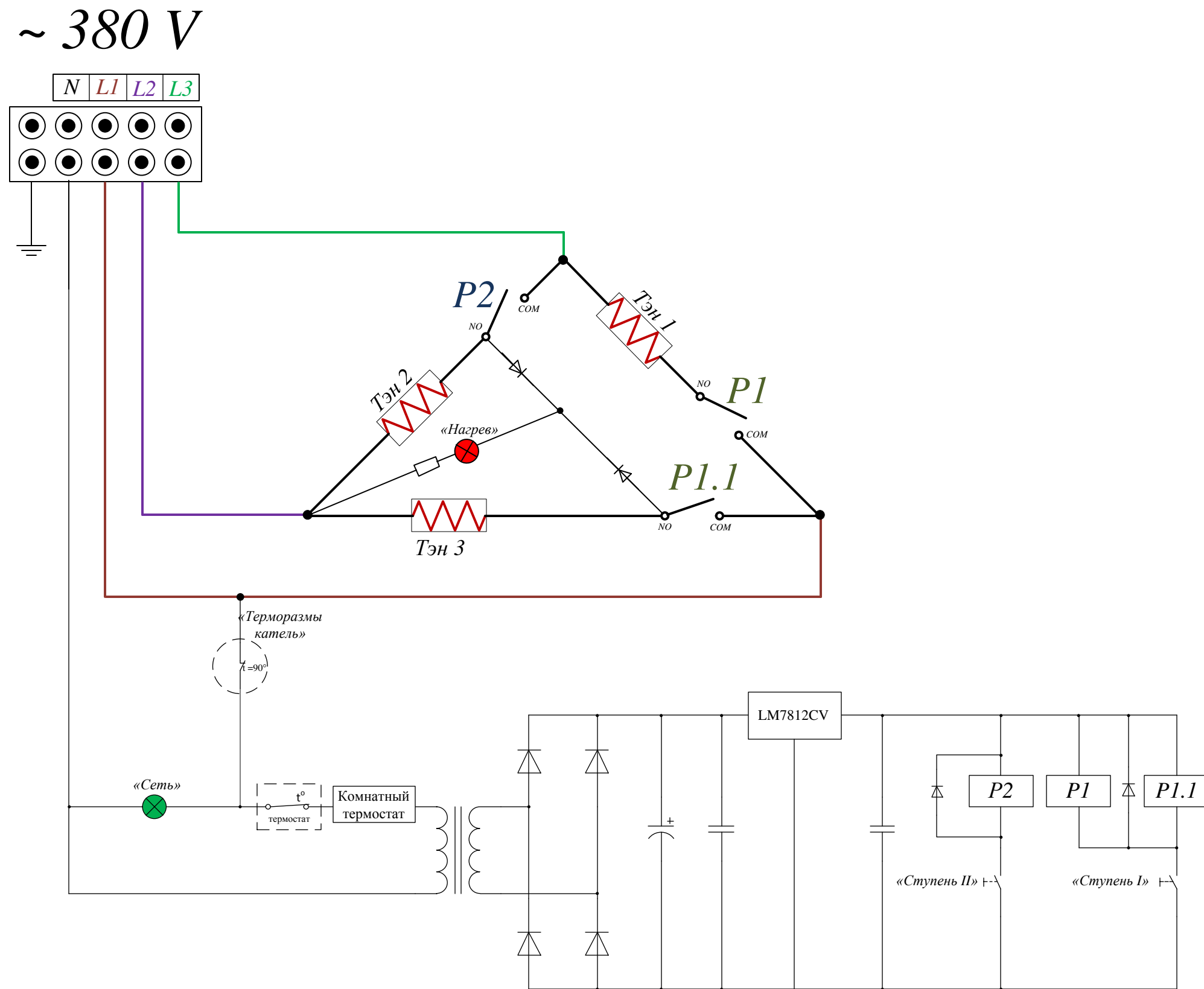
Рисунок 1 – Схема электрическая принципиальная для котлов «Есопот» 12, 15 кВт на 380 В
