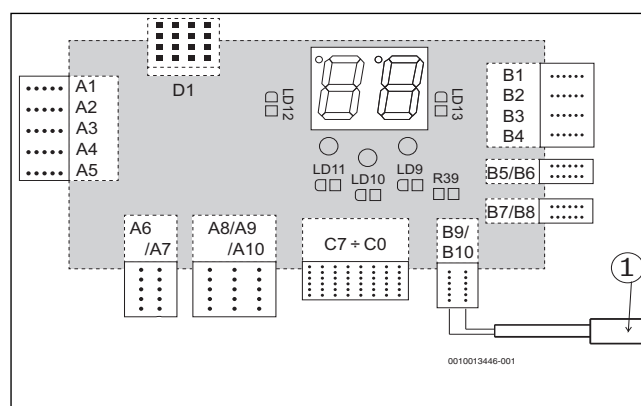
Obr. 1 Pripojenie snímača k svorkám B9/B10
