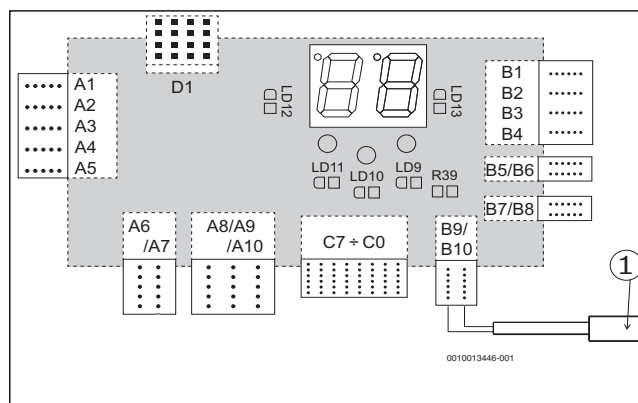
Сурет 1 Датчикті клеммаларға жалғау B9/B10
