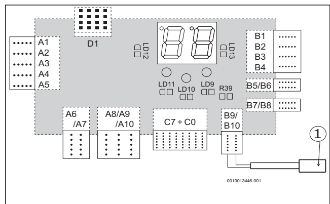
Мал. 1 Під'єднання датчика до клем B9/B10
