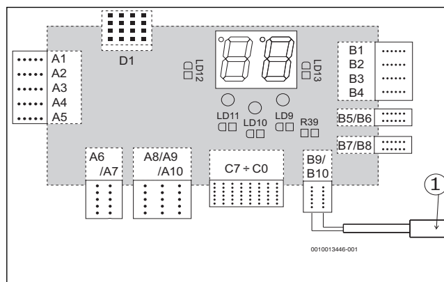
Fig. 1 Raccordement de la sonde aux bornes B9/B10
