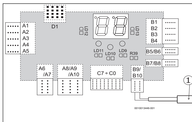
Sl. 1 Priključak osjetnika na stezaljke B9/B10
