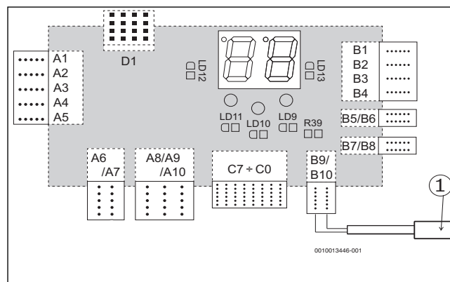
Sl.1 Priključitev tipala na sponki B9/B10
