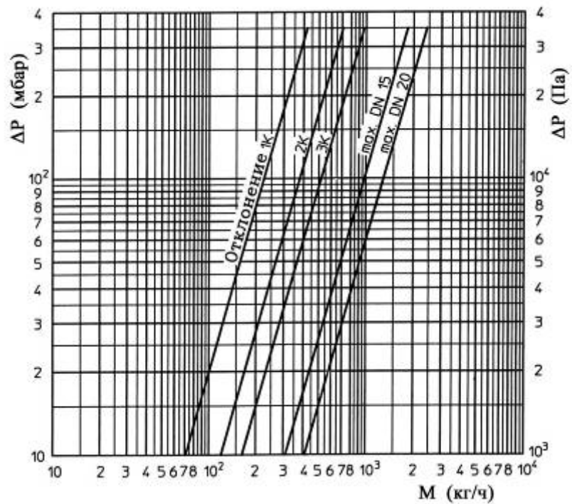
Рис. 3.3. Гидравлические характеристики термостатов фирмы «Овентроп»: а – AV6 для двухтрубных систем отопления; б – M для однотрубных систем отопления
