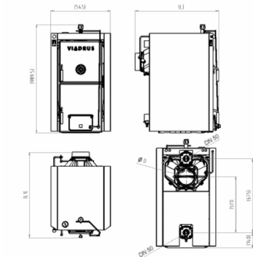
Рис.№ 12 Присоединительные размеры котла VIADRUS HERCULES U 22 без коробки управления
