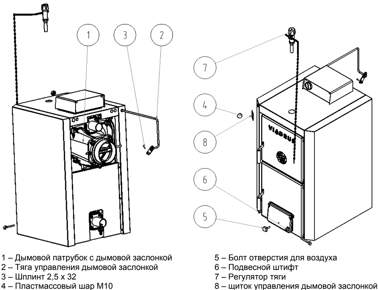
Рис. № 23 Управление дымовой заслонкой
