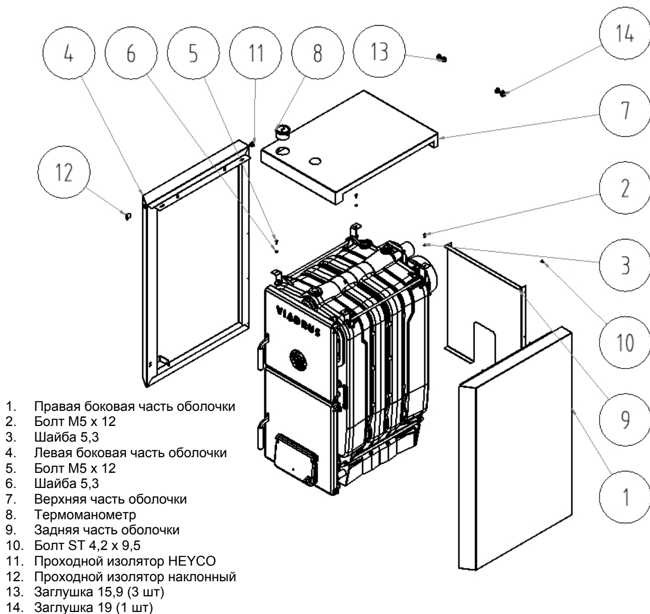
Рис. № 19 Состав оболочки котла без коробки управления
