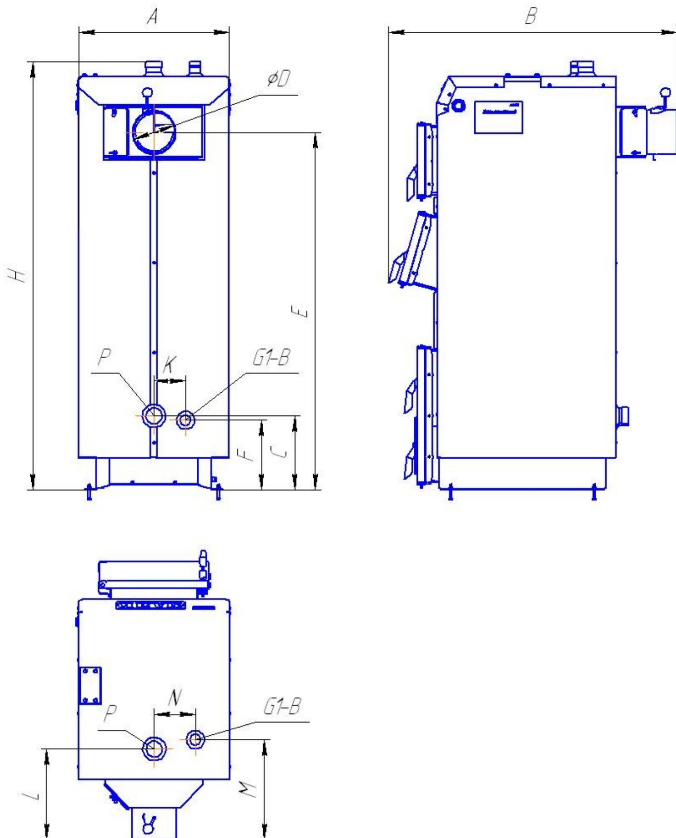
Рисунок 3. Приєднувальні розміри
