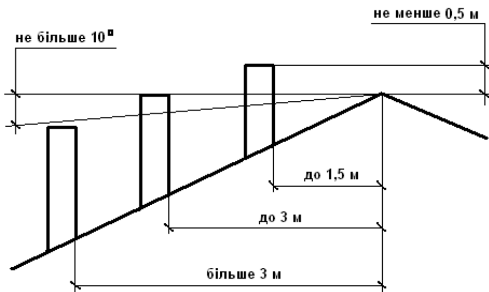
Рисунок 5. Розміщення димоходу
