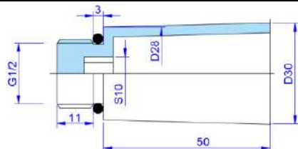
ВТр.792.М Комплект длинных монтажных пробок
