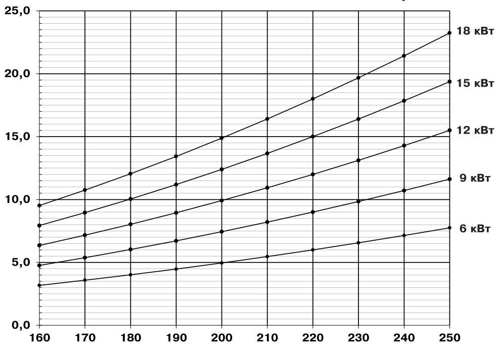
Рис.8 График изменения мощности миникотельной в зависимости от питающего напряжения
