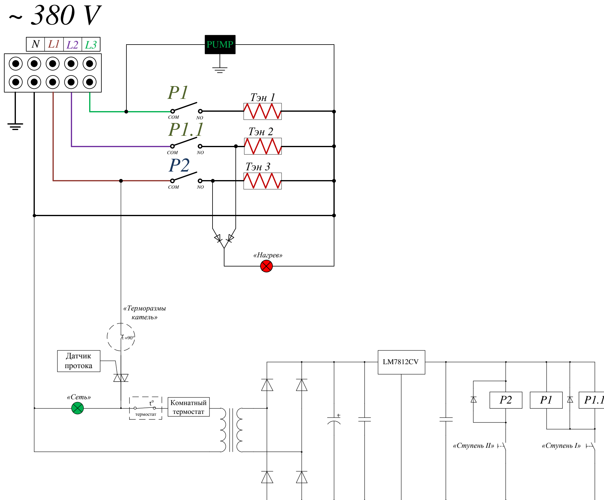
Рисунок 2 – Схема электрическая принципиальная для котлов «Standart» на 380 В
