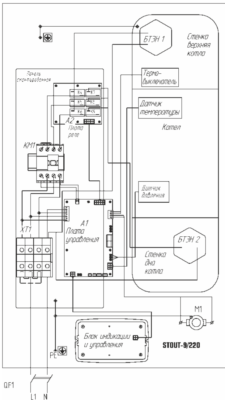
Рисунок 13 Схема подключения SEB-0001-00009 к сети 220 В.
