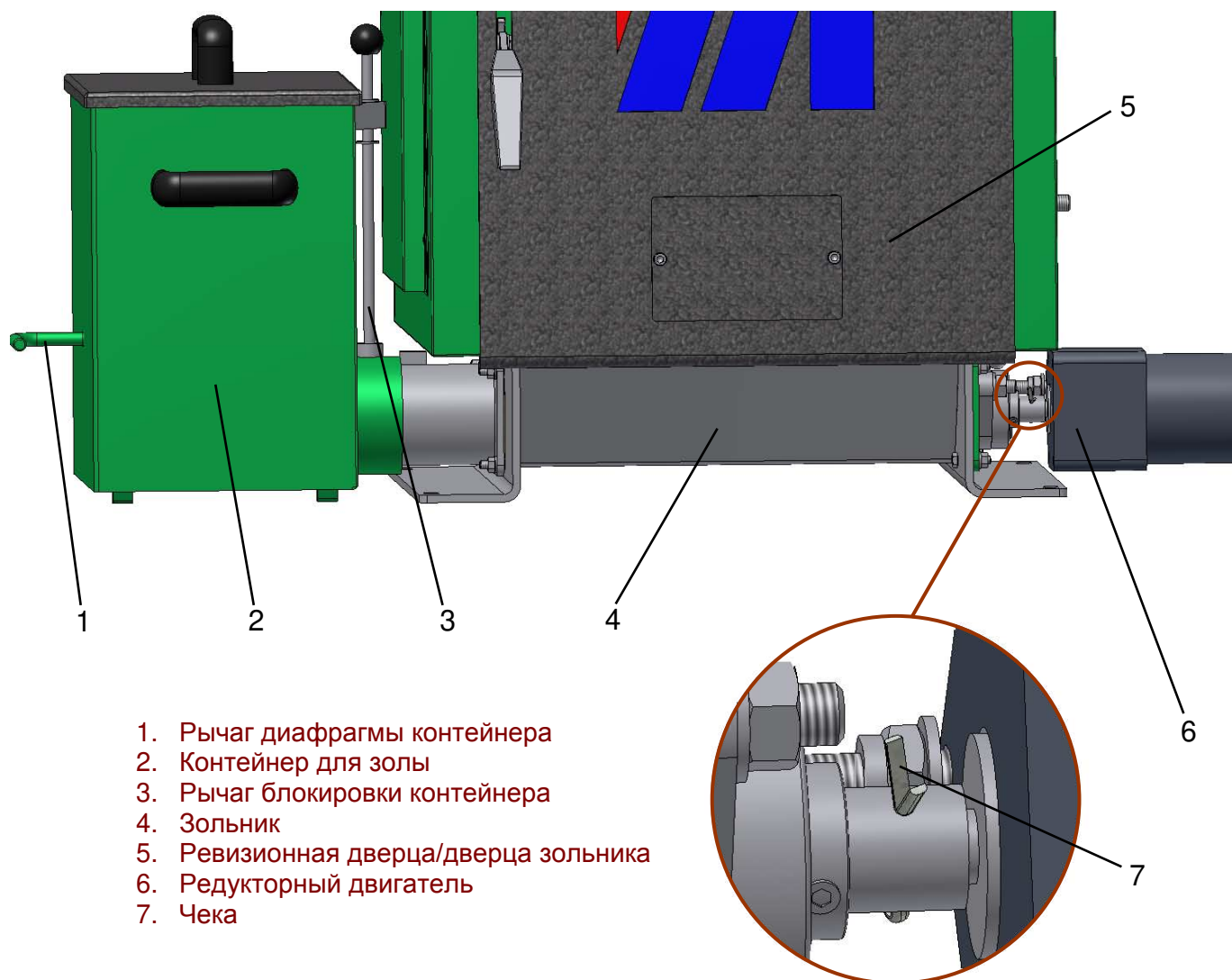
Рис. 4. Внешний вид теплообменника Vento Bio (Eko) с системой удаления золы.
