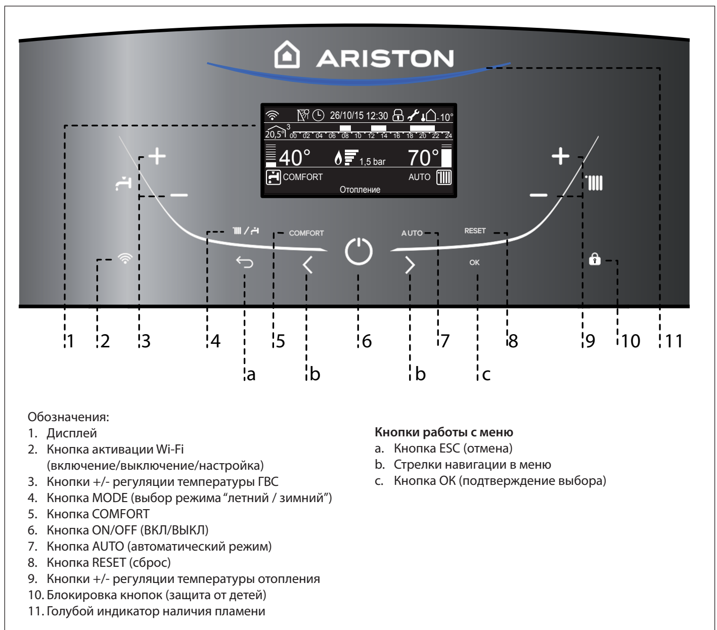
Панель управления
