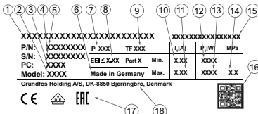
Рис. 2 Пример фирменной таблички MAGNA3
