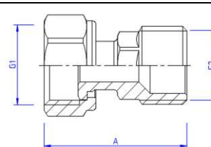
VTr. 613 Соединитель с накидной гайкой В-Н
