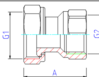
VTr. 614 Соединитель с накидной гайкой В-В
