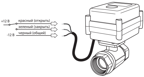
Рис. 2 Электрическая схема подключения крана с электроприводом серии Neptun AquaControl 12B
