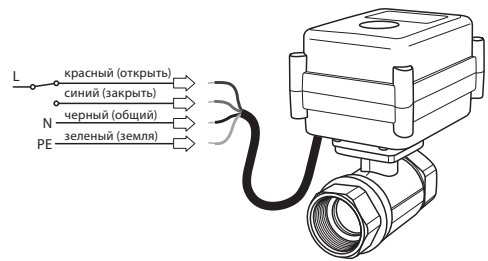
Рис. 1 Электрическая схема подключения крана с электроприводом серии Neptun AquaControl 220B
