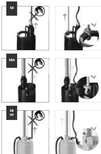
Рис. 3 Подъём насоса
